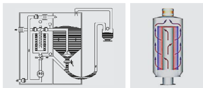
balra: RDM működési sémavázlat „szárazlevegős” anyagszállítási opcióval jobbra: SOMOS® egykamrás-szárítóközeg tartálykialakítás a szárítóközeg optimalizáltan hatékony felhasználása érdekében - a szárítóanyag gyors és hatékony regenerációja költségmegtakarítást eredményez.
